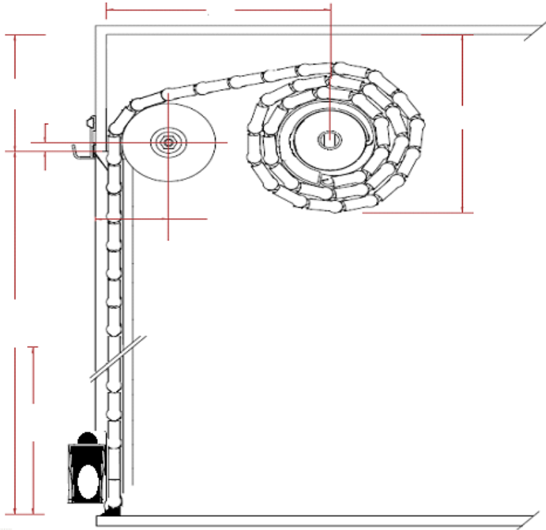
Монтажная схема
